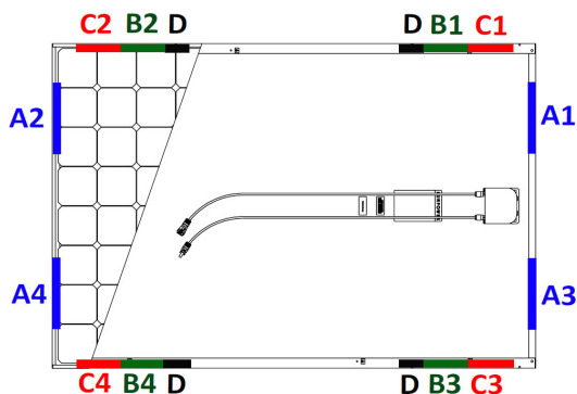
Abbildung 2: Befestigungszone für Sunpower Module
