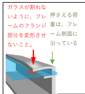
図 1a: クランプで押える荷重の位置
