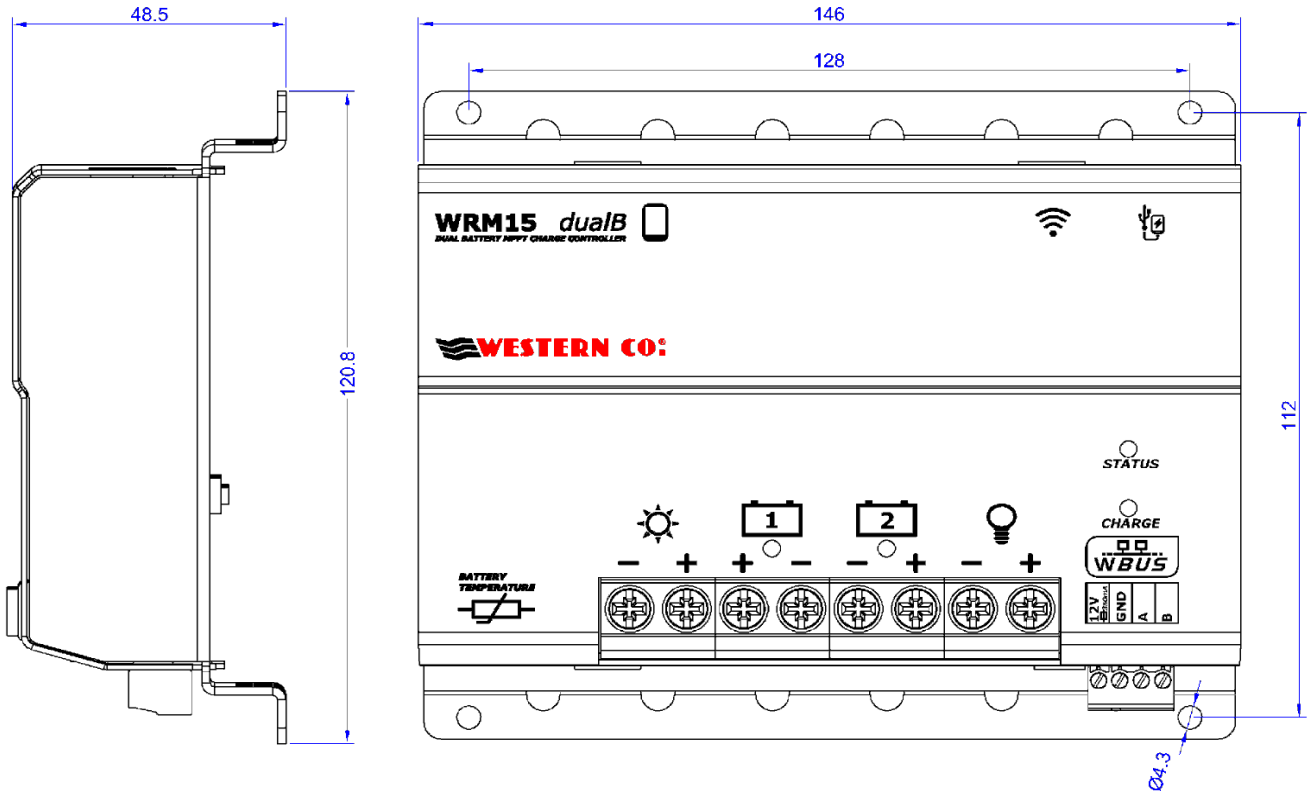
Fig. 5 Dimensioni (mm)
