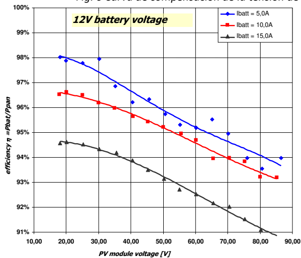
Fig. 7 Rendimiento del WRM15 dualB/dualB-E en función de la tensión de panel para sistema de 12 V y 24 V
