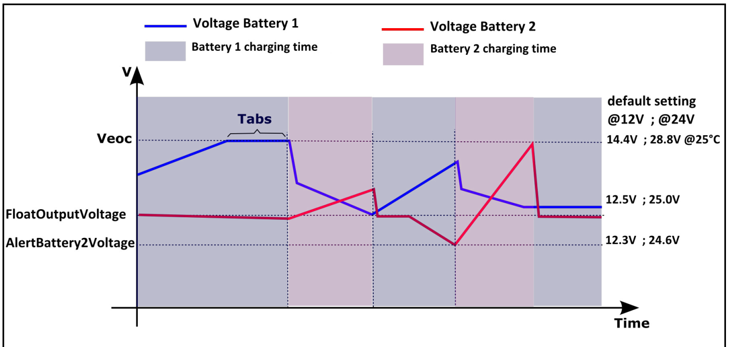
Abb.3 Steuerung Batterie 1 und Batterie 2
