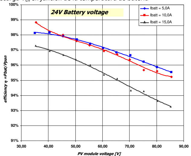
Fig. 7 Rendimiento del WRM15 dualB/dualB-E en función de la tensión de panel para sistema de 12 V y 24 V
