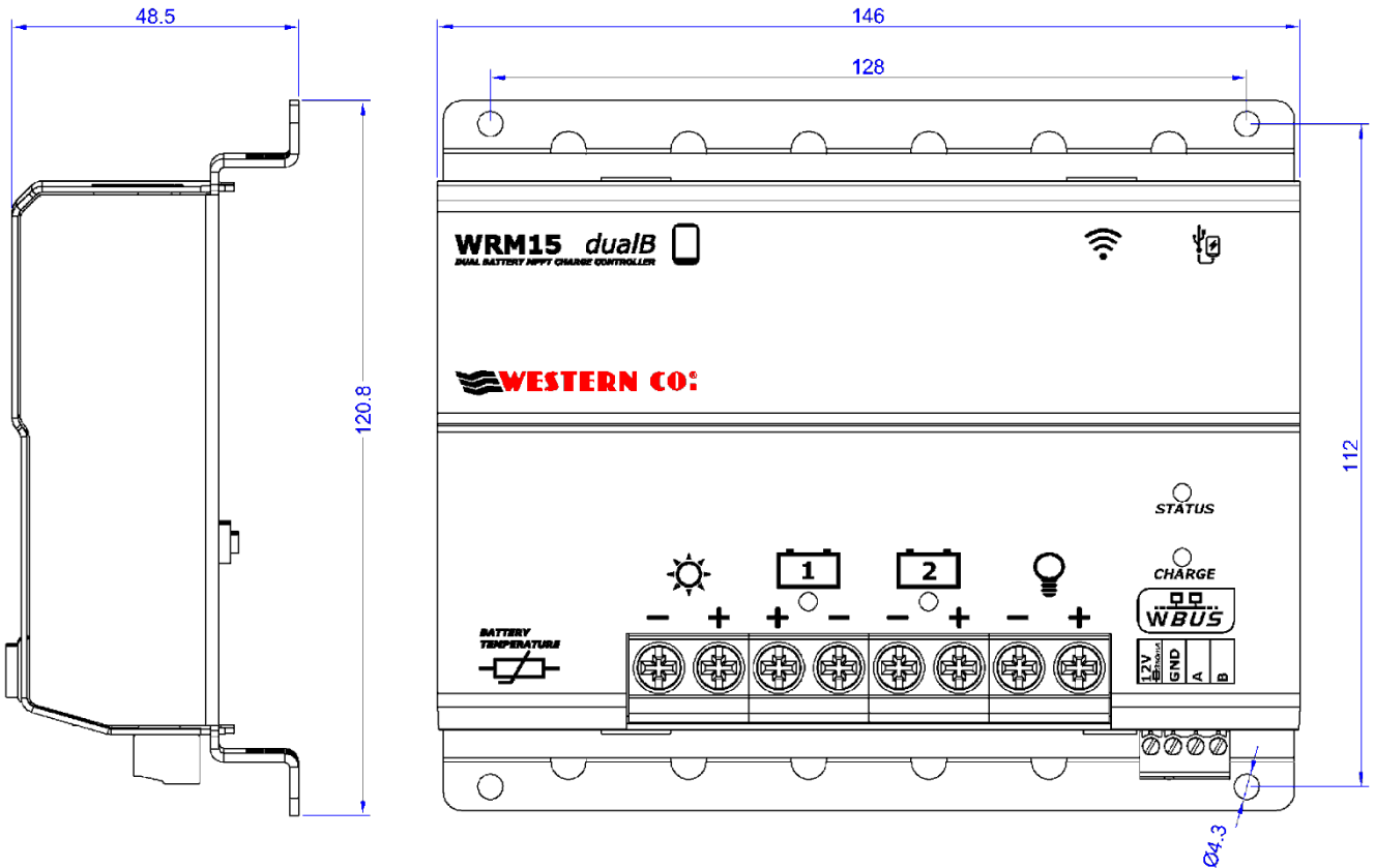
Fig. 5 Dimesions (mm)
