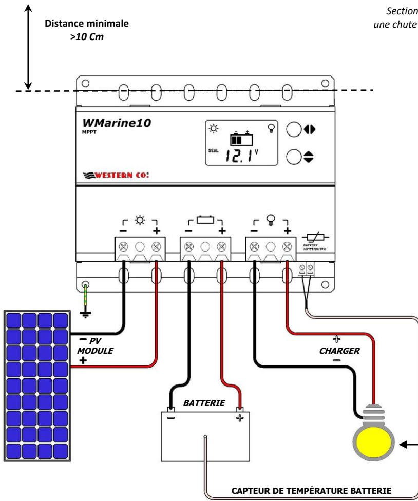
Fig.2 Schéma de branchement
