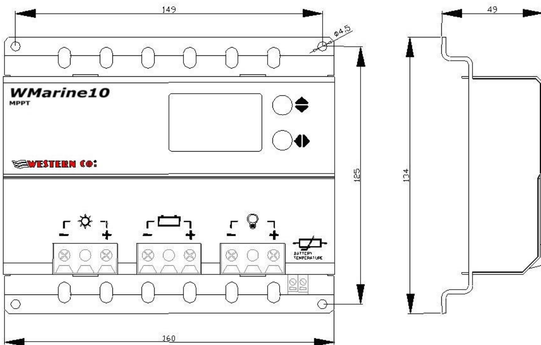
Fig.4 Dimensioni
