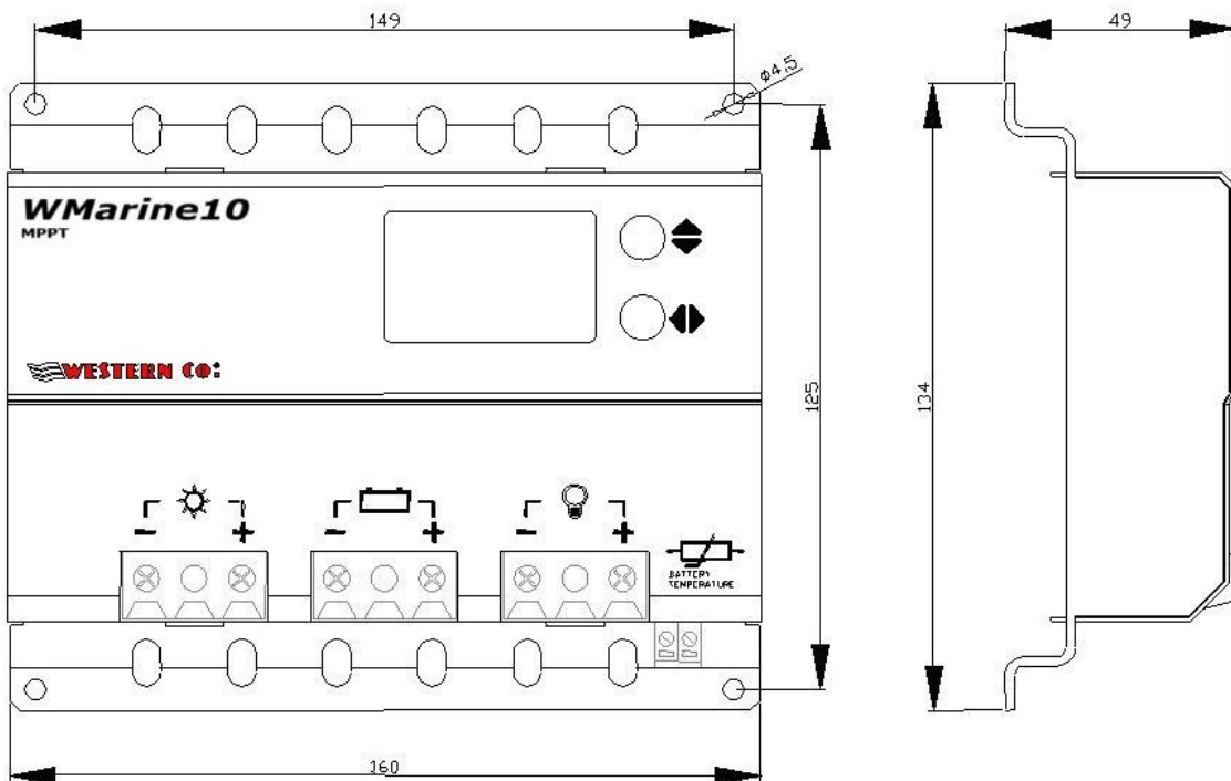
Fig.4 Dimensiones
