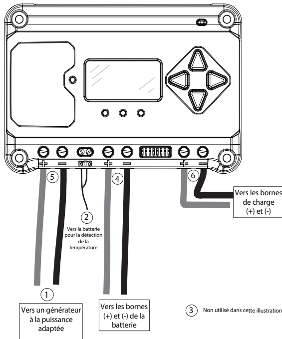
Figure 3-2. Raccordement de l'EcoPulse
