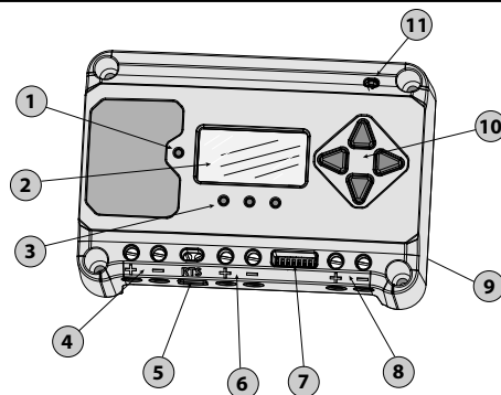
Figure 2.1. Caractéristiques de l'EcoPulse
