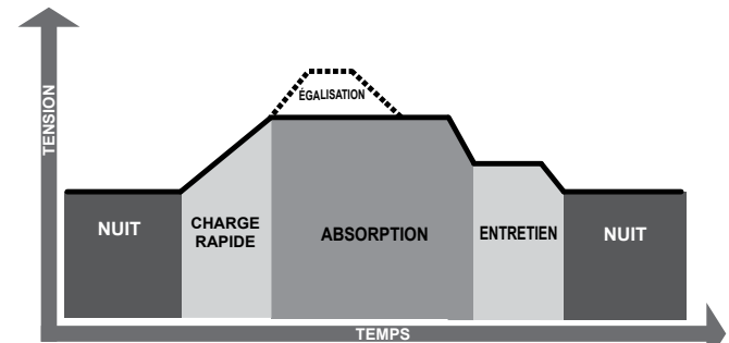
Figure 4.1. Algorithme de charge de l'EcoPulse
