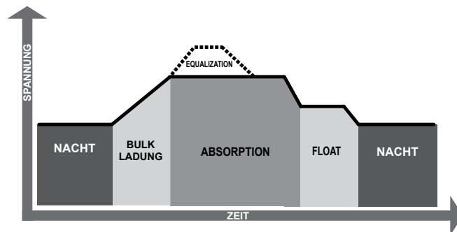
Abbildung 4.1 – EcoPulse Ladealgorithmus
